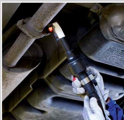
Ruostuneiden ja jumittuneiden liitosten lämmitys alustassa ja pakoputkessa
